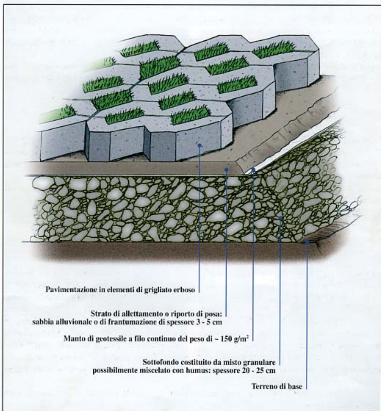
Fig. 2 - Schema di posa della pavimentazione in grigliato erboso
