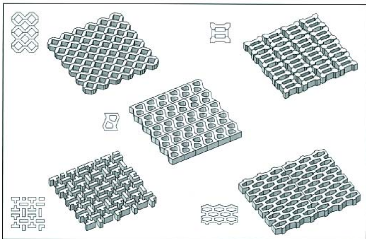
Fig. 1 - Elementi grigliati in calcestruzzo per pavimentazioni erbose più diffusi
